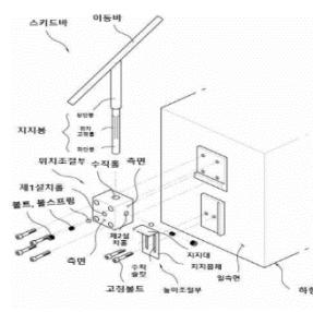
<원터치 세팅용 스키드바 장치>
